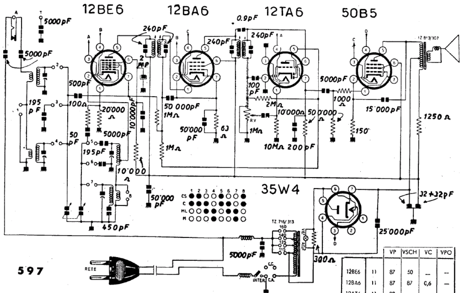
PHONOLA RADIO - Mod. 597 - Medie da 585 a 430 M e da 450 a 190 m; corte da 50 a 37 e da 58 a 16 m. MF a 470 kc. Consumo 30 watt. Potenza 1,2 W.
